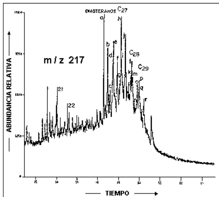
Distribución de biomarcadores esteranos m/z del Mene Pozón (Tomado de: Del Olio, 1993)
