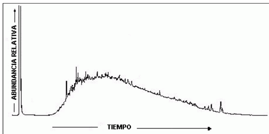
Cromatograma de la fracción saturada del Mene de Pozón (Tomado de: Del Olio, 1993)
